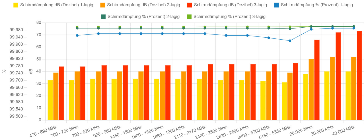
Schirmdämpfung - HiFreq-Standard-Powder - 4 m 2 pro Liter - 470 MHz bis 40.000 MHz (40,0 GHz)
