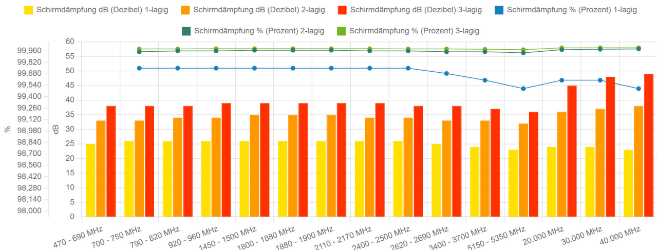
Schirmdämpfung - HiFreq-Standard-Powder - 8 m 2 pro Liter - 470 MHz bis 40.000 MHz (40,0 GHz)
